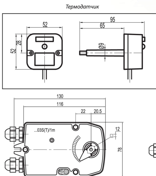
РАЗМЕРЫ мм
