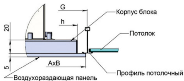
Узел примыкания панелей к профилю
