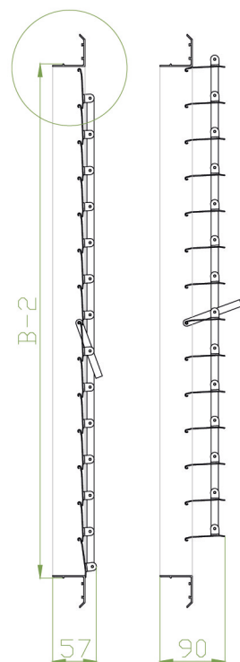
ФВР2Р ручка спереди
