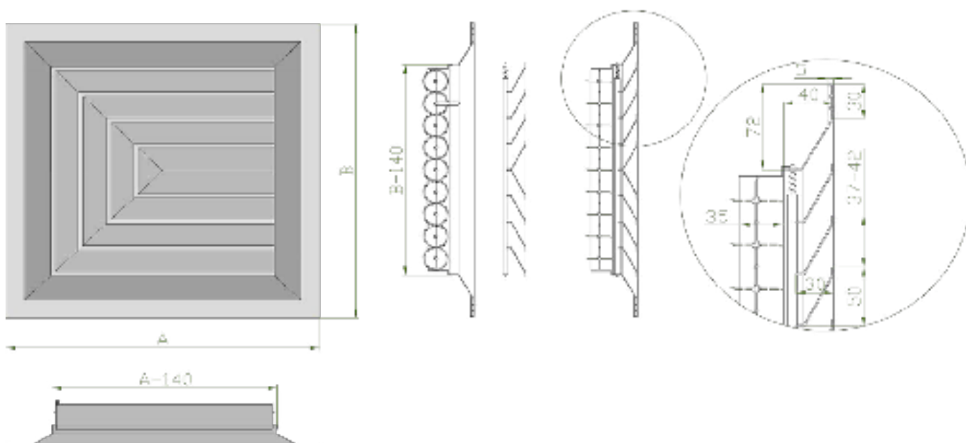
Габаритно-посадочные размеры потолочной решетки с клапаном расхода воздуха ЗАРР-Р A \times B габаритные размеры решетки
