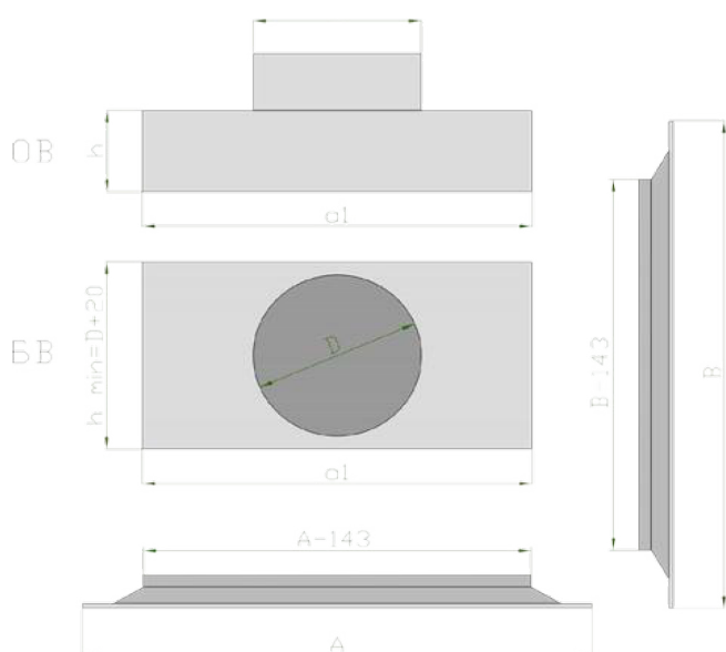
Установочный размер адаптера для стандартных типоразмеров потолочных решеток
