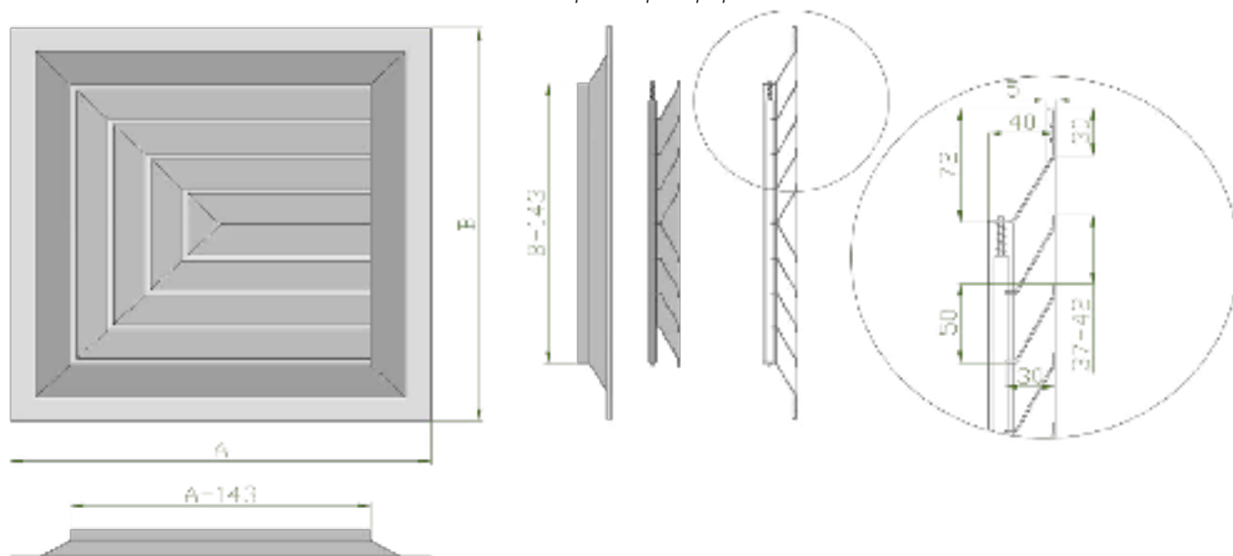
Габаритно-посадочные размеры потолочной решетки ЗАРР A \times B габаритные размеры решетки
