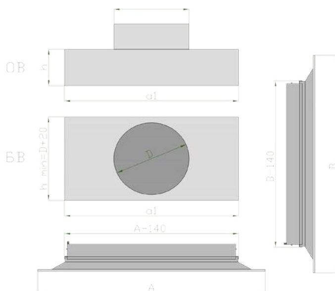
Установочный размер адаптера для стандартных типоразмеров потолочных решеток
