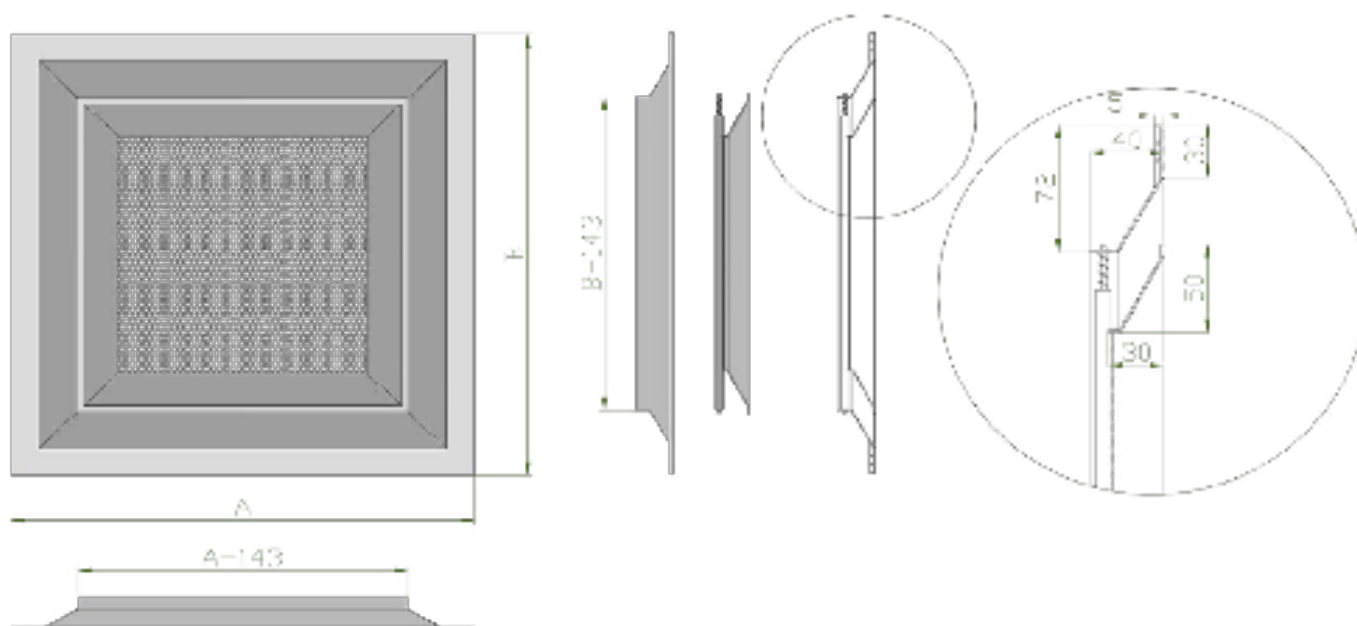
Габаритно-посадочные размеры потолочной решетки 1APR АхВ габаритные размеры решетки
