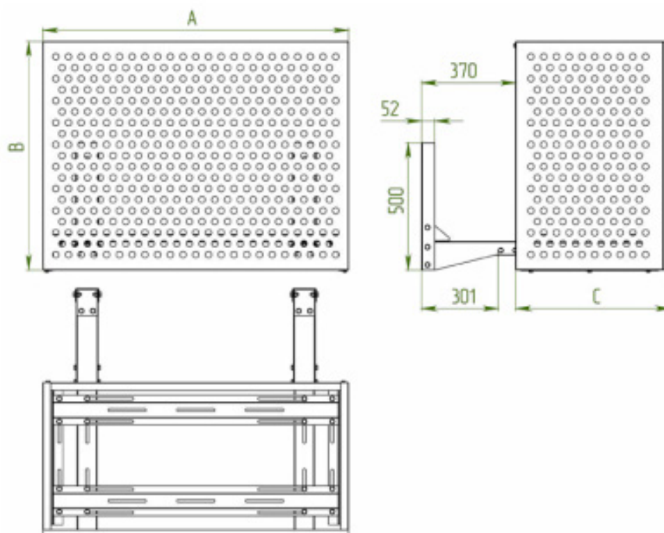
Корзина с кронштейном AKFU
