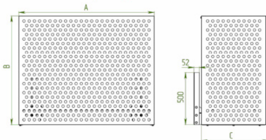
Корзина с кронштейном AKF
