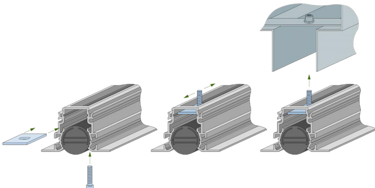
Монтаж щелевого диффузора SL35
