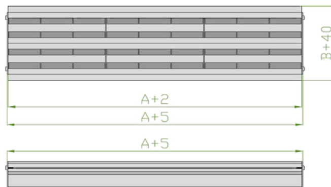
E2 Концевая секция с одной заглушкой
