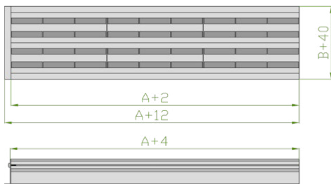
E1 Концевая секция с одним фланцем
