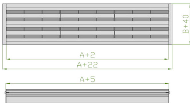
F1 Одиночная секция с фланцами
