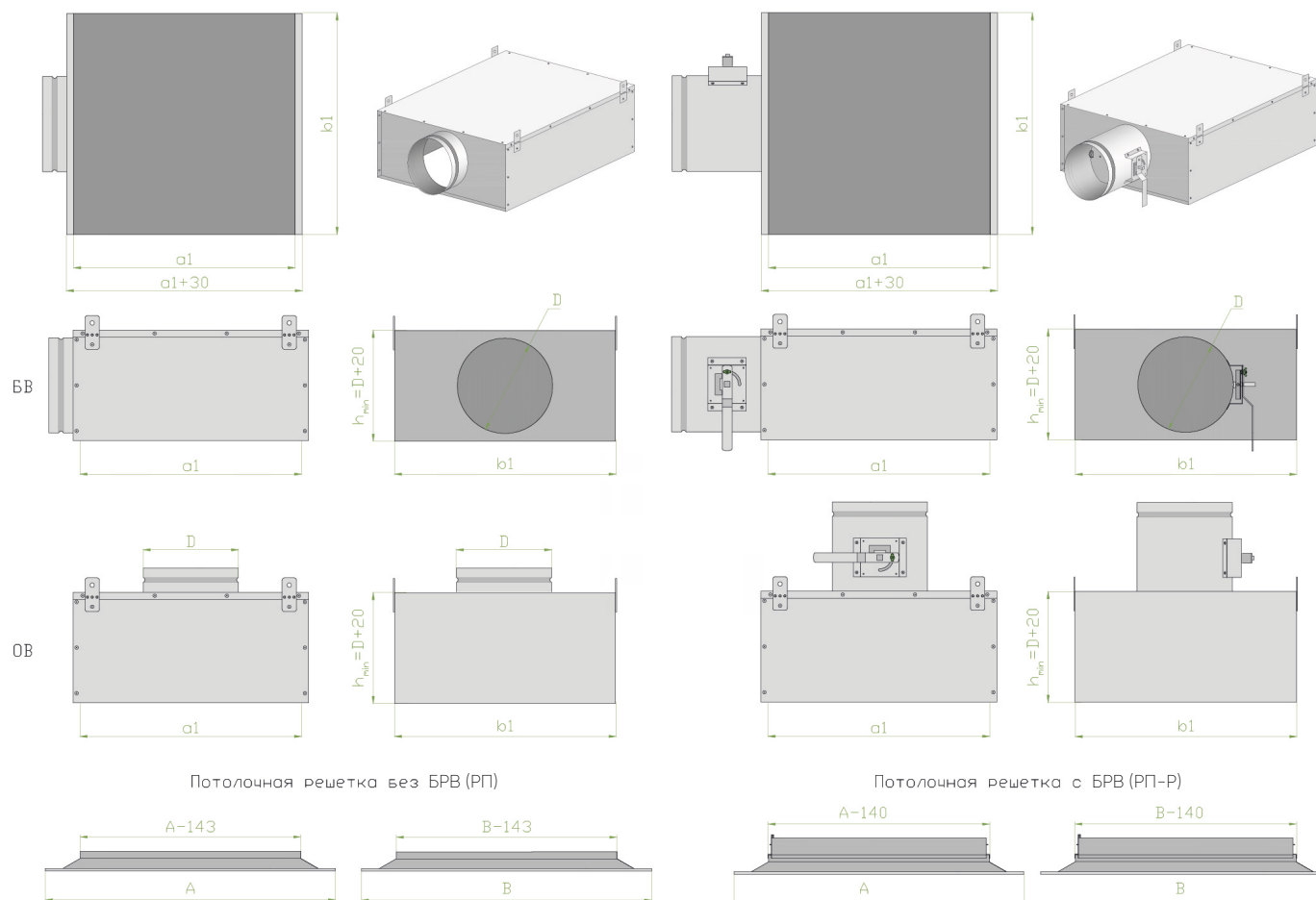
Камера статического давления КСД (без дроссель-клапана)
