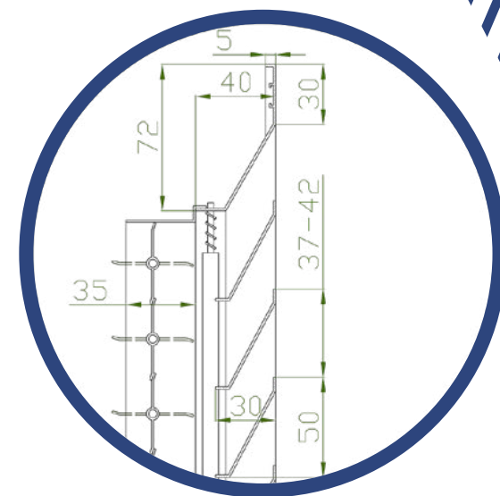
Габаритно-посадочные размеры потолочной решетки с клапаном расхода воздуха 2РП-Р АхВ габаритные размеры решетки
