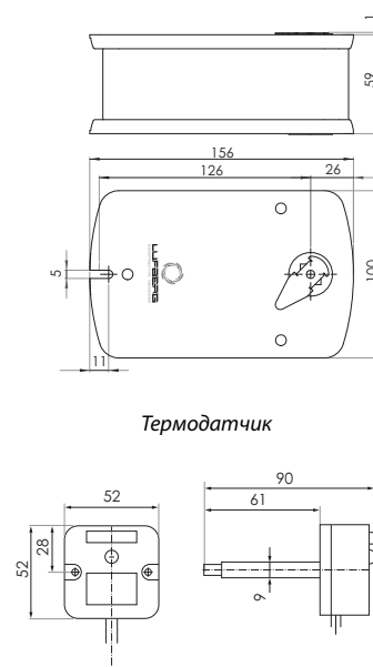
РАЗМЕРЫ (мм)
